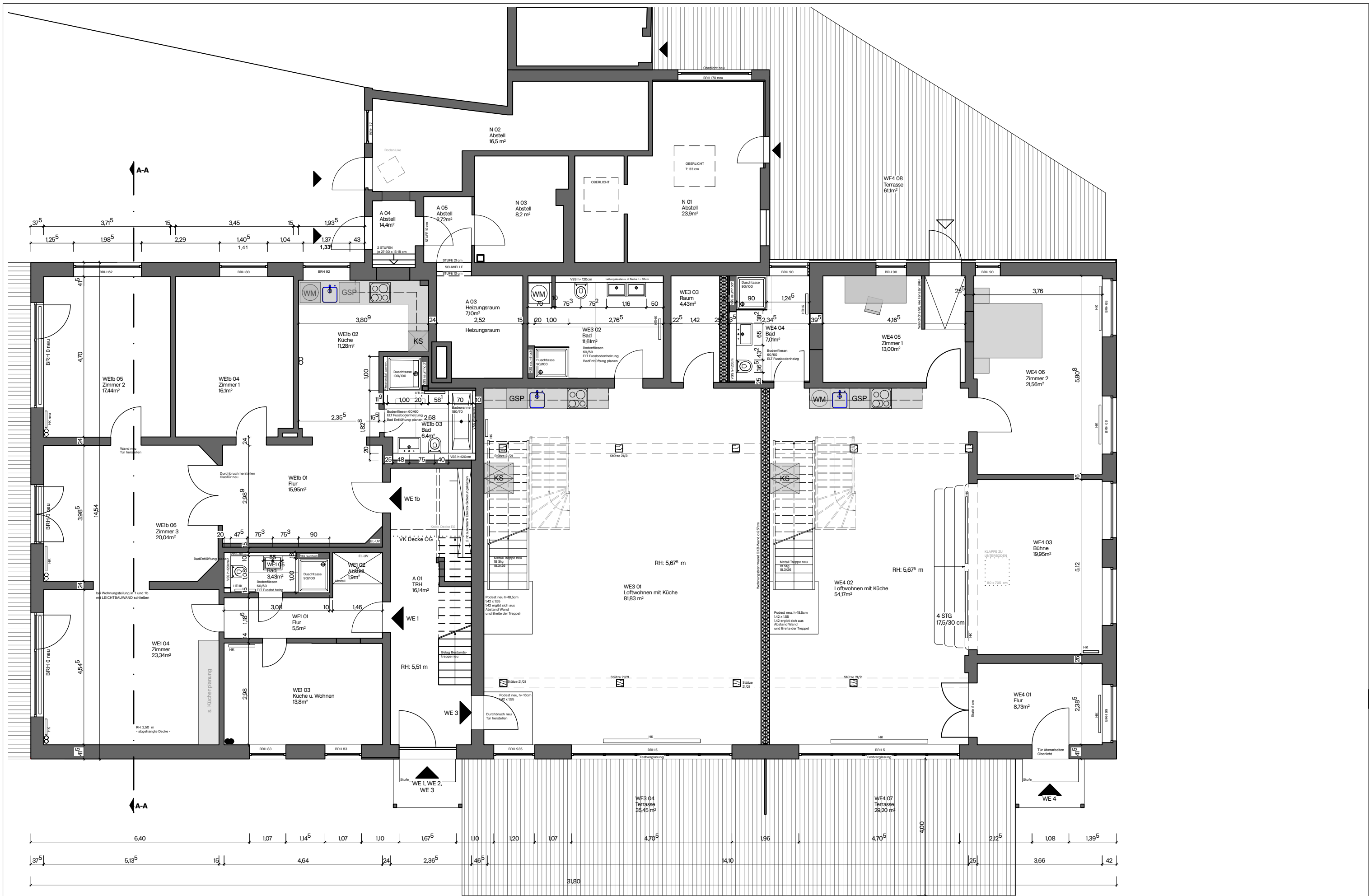
Erdgeschoss Grundriss
